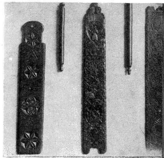
I. Eiken mangelplank uit Friesland. II. Mangelplank van 1672. III. Mangelplank uit Noord-Holland. Hiertussen twee rollen.
